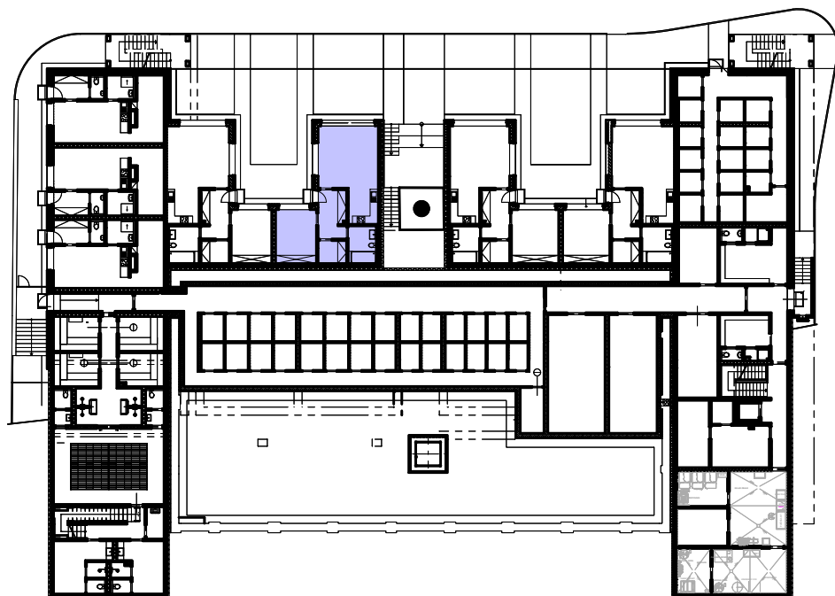
Schéma půdorys
